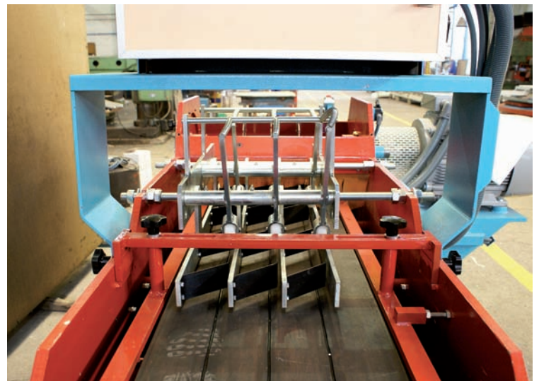
Detalle Guías
